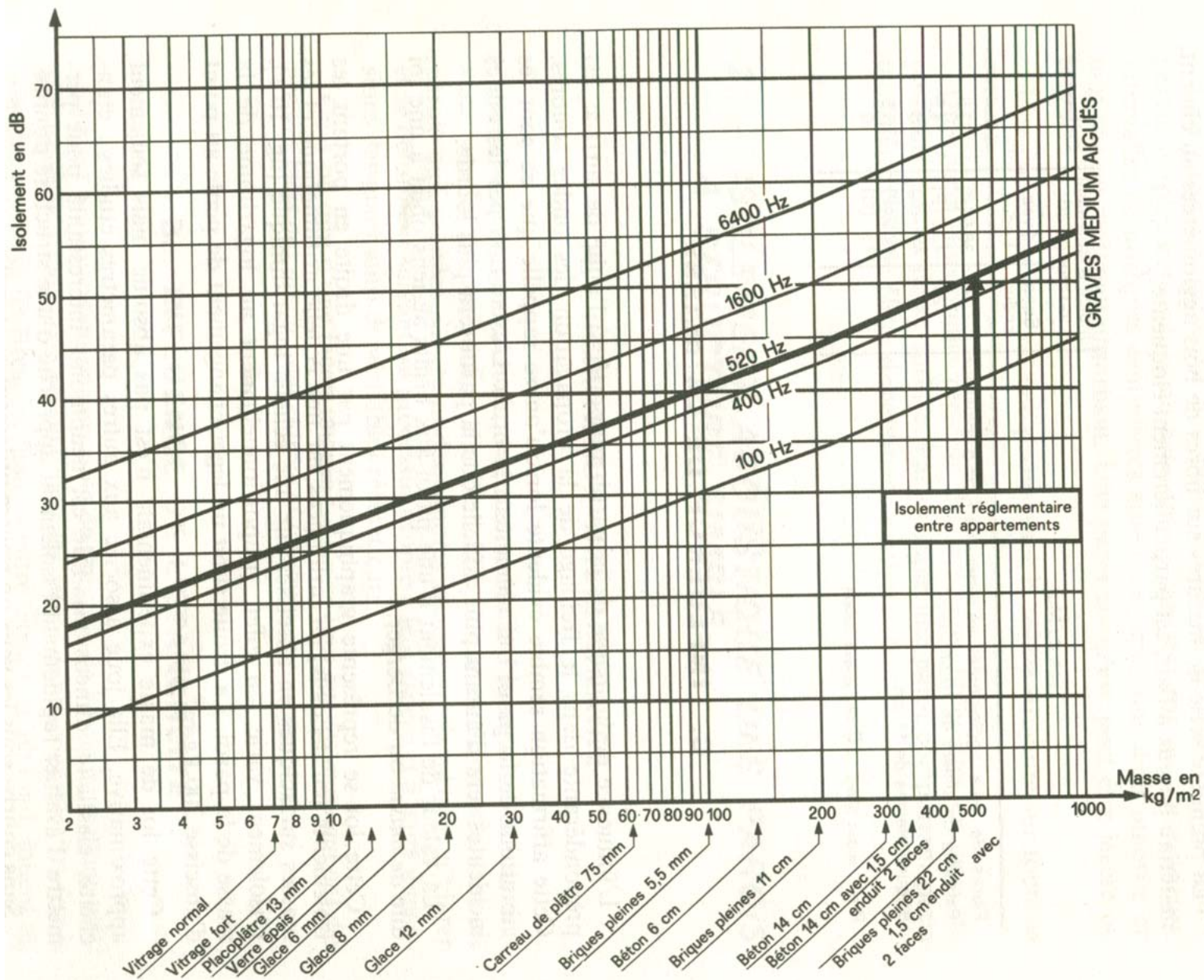
Abaque de la loi de masse
